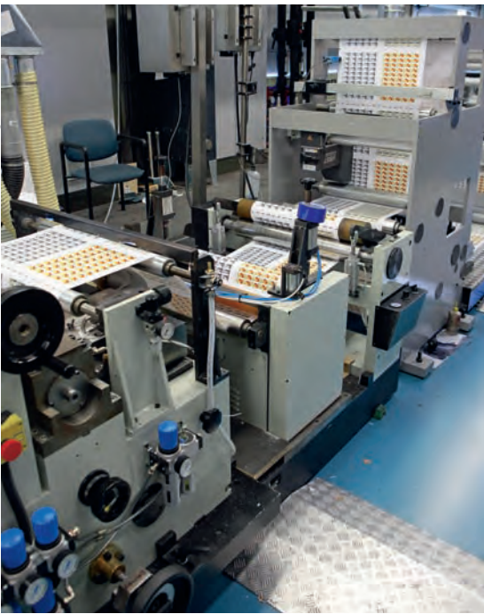
Op de rotatiepersen rollen postzegelvellen op rol of op vel van de machine.
