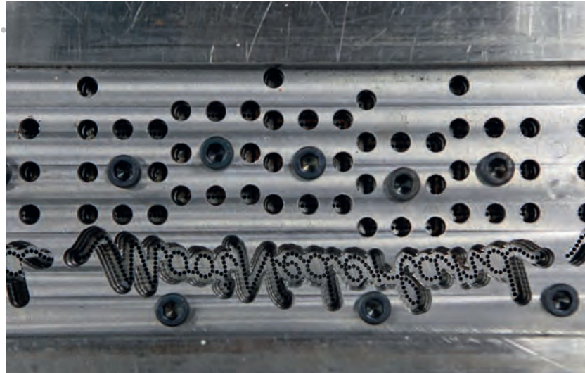
Met een perforieerkam worden de postzegelvellen geperforeerd. De kam op deze foto is speciaal vervaardigd voor de serie Mooi Nederland.
